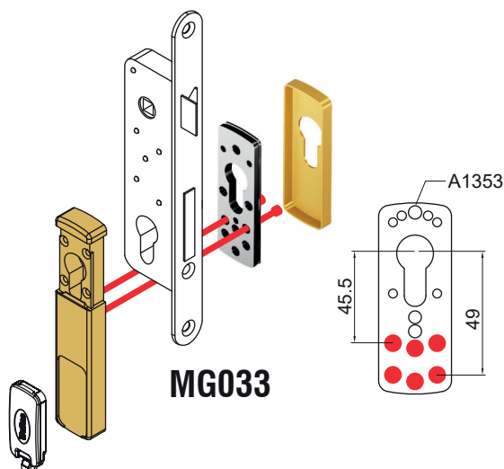
MG033 X ASSA ABLOY DIN 18250 X ADAMS RITE
