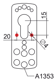
MG033 X ASSA ABLOY DIN 18250 X ADAMS RITE
