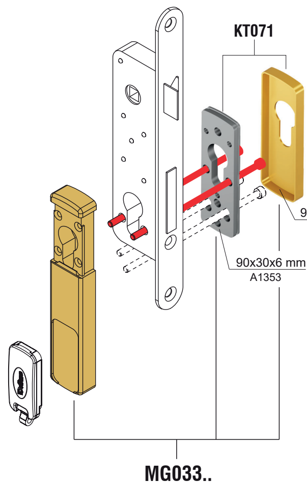
MG033 X CISA serie 16 / 46
