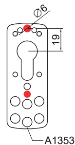
MG033 X ISEO - MULTIBLINDO
