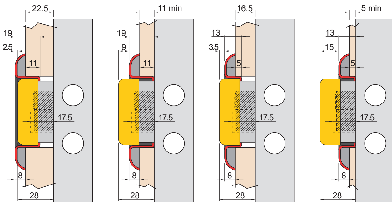
KM0P3G CHIAVE MAGNETICA MAGNETIC KEY
