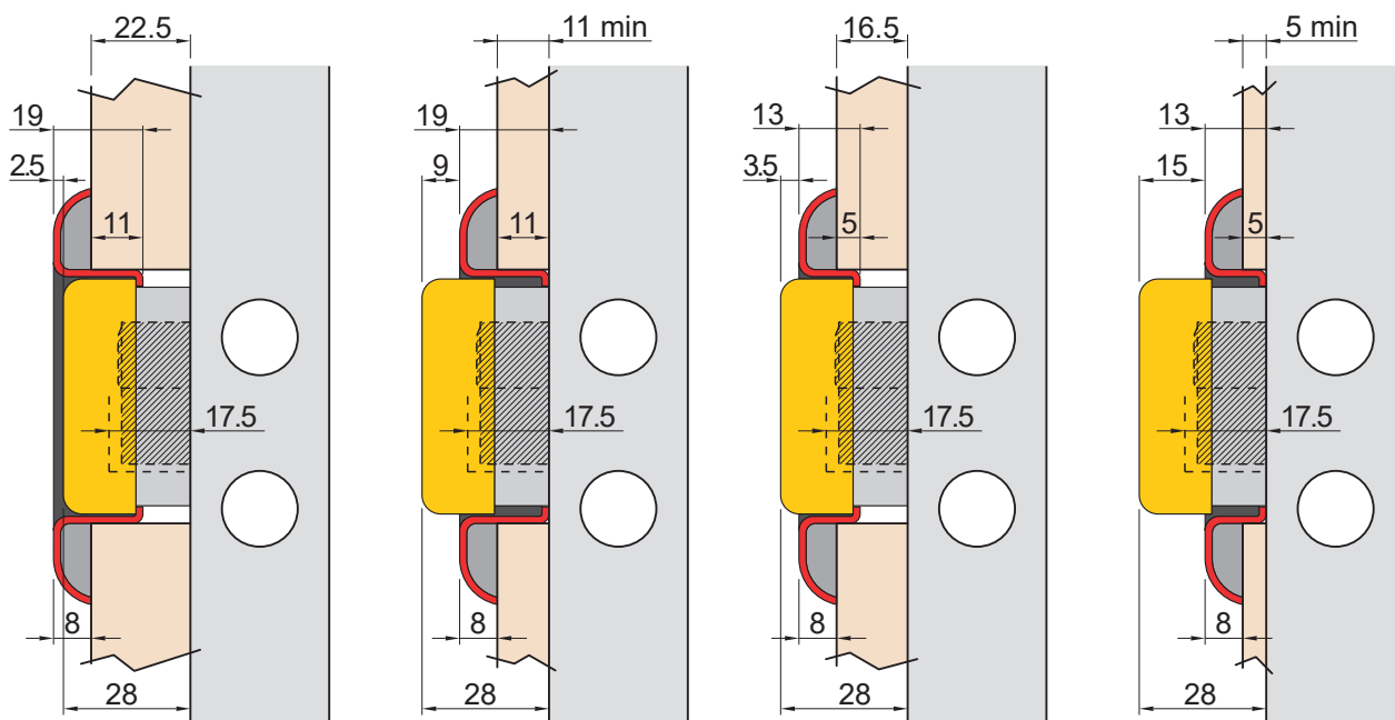
KM0P49 CHIAVE MAGNETICA MAGNETIC KEY
