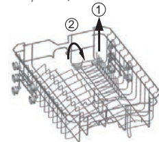
Coșul superior
