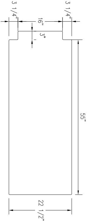
CUTOUT TEMPLATE
