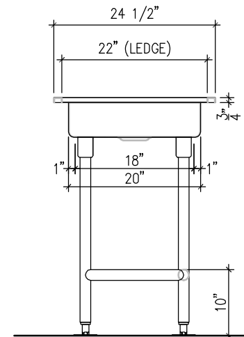
SIDE ELEVATION SCALE: 2" = 1'-0"
