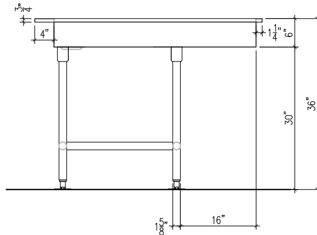
FRONT ELEVATION SCALE: 2" = 1'-0"
