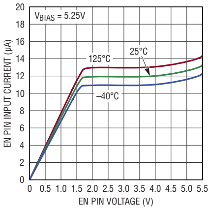
EN Pin Input Current
