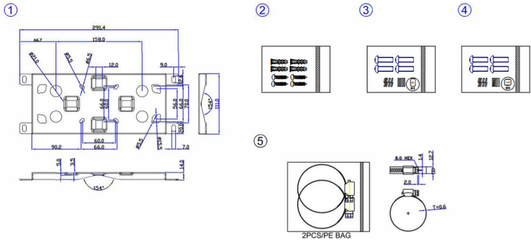
GTT-MNT-LP1S (SUS304)
