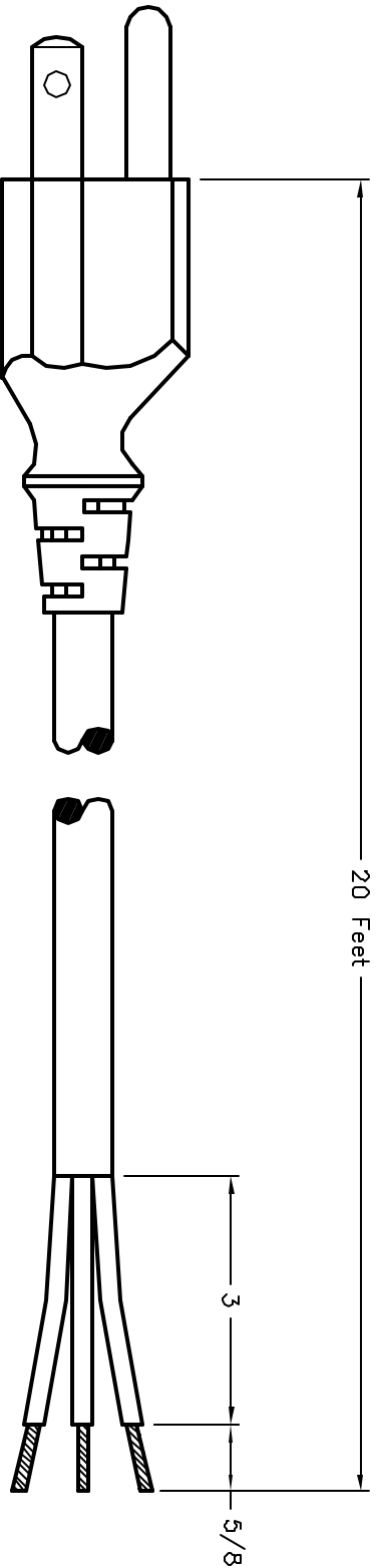
NEMA 5-15P
