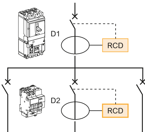
D1 and D2 in series.
