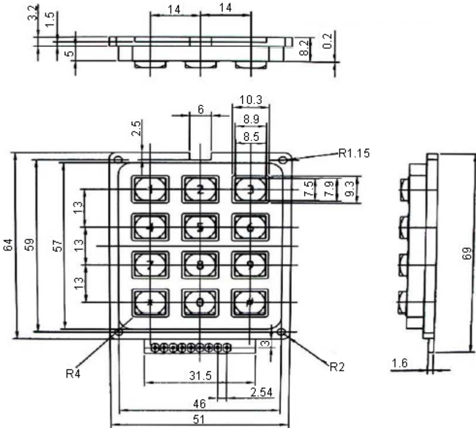
Dimensions : Millimetres
