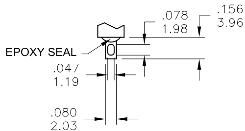
SOLDER LUG
