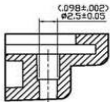
△ A-A SECTION
