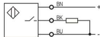
PNP NO
