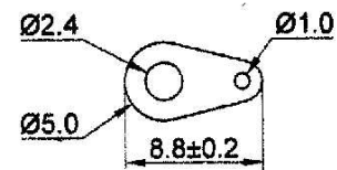
SOLDER LUG
