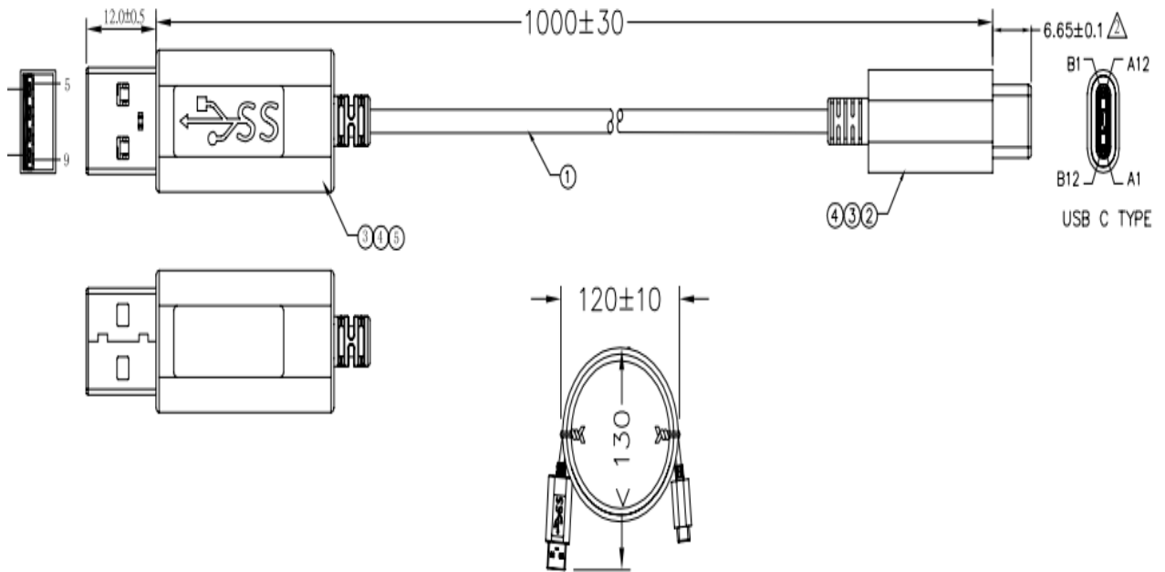
扎線圖
