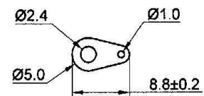
SOLDER LUG
