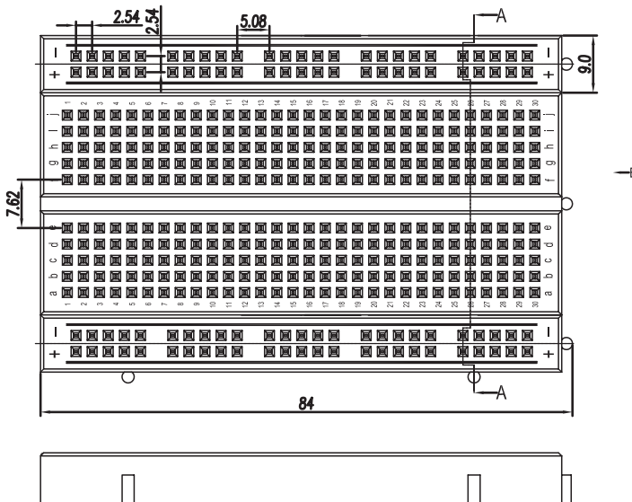
Dimensions : Millimetres
