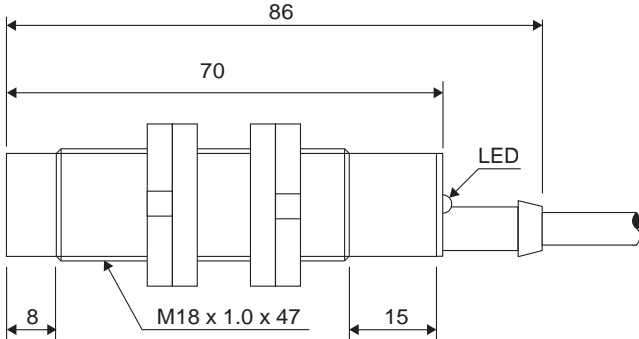
Fig. 7 Cable 2377238
