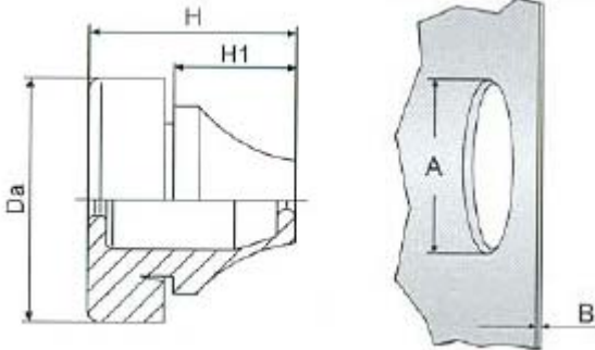
Dimensions : Millimetres
