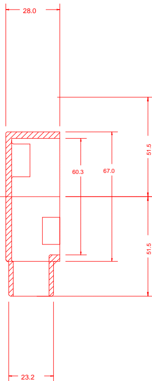
SECTION A-A
