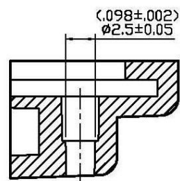
△ A-A SECTION
