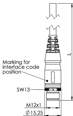
Dimensions : Millimetres
