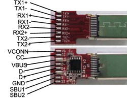
P2 频位示意图:
