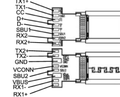
P2 频位示意图:
