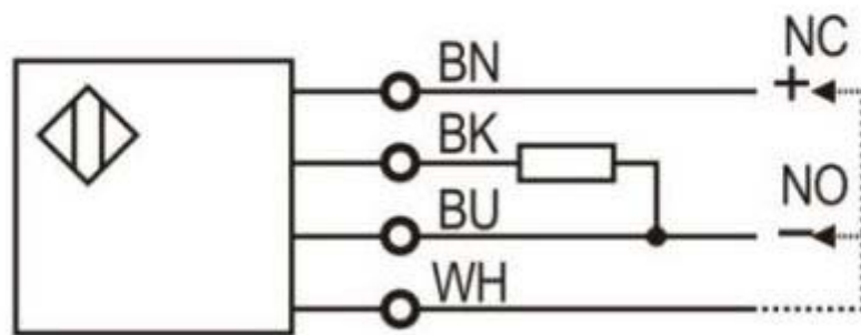
PNP NO/NC
