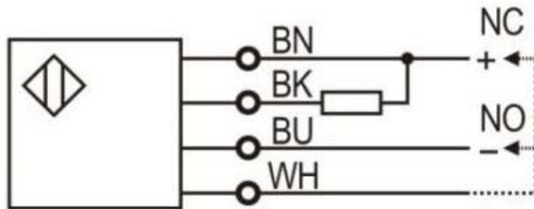
NPN NO/NC
