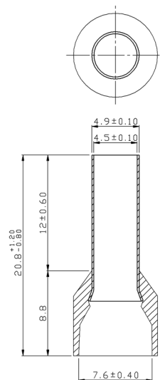
Dimensions : Millimetres
