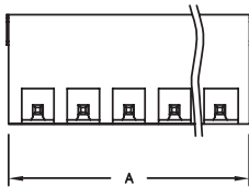
Dimensions : Millimetres
