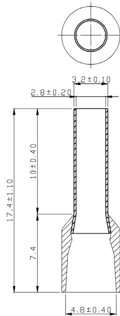
Dimensions : Millimetres
