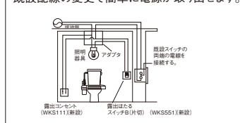
ⓂWG4390※ 希望小売価格 4,100円(税抜) 丸型引掛シーリングアダプタ (増設電源端子付)6A 125V
