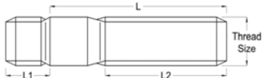
DIN 938
