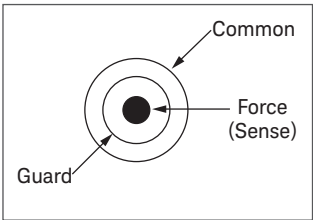
Figure 3.4. SMU terminal
