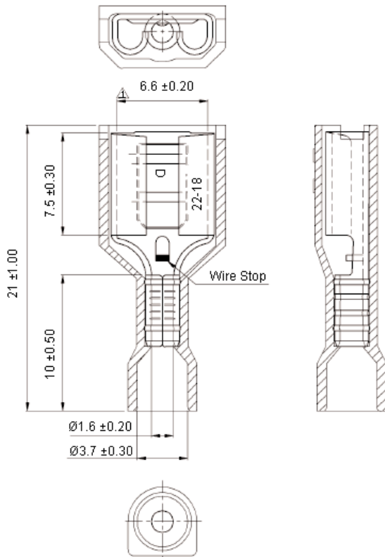
Dimensions : Millimeters
