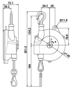
SB-3K/5K SB-7K(S)
