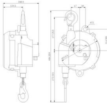
SB-40K / SB-50K
