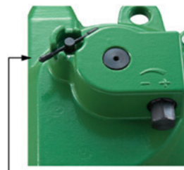
Lock Spring Drum Position 鎖住螺旋座位置
