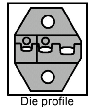
Die profile
