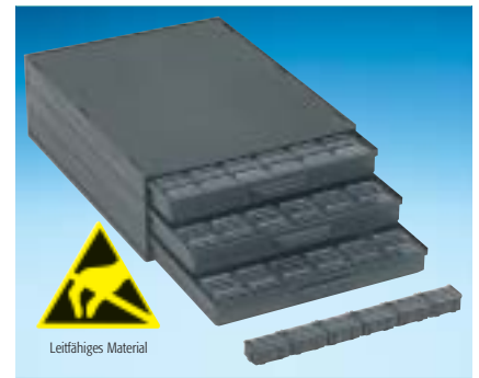
Art.-Nr. SMD-Schrank A 1-4 ESD 72 Schrank mit 3 Schubladen inkl. 3 x 72 = 216 Stück
