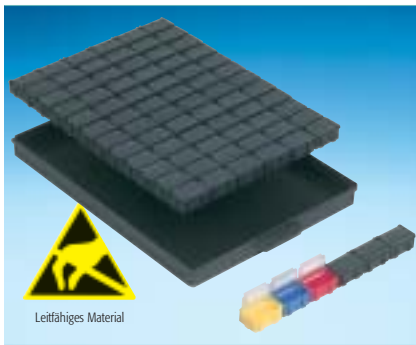
Art.-Nr. 72 SMD-Boxen N2 genau passend in A 1-4/16-6-10 Innenmaß 340 x 250 x 22
