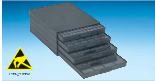
Art.-Nr. A 1-4/4 ESD MIX Leitfähiger Schrank mit 4 Schubladen, je Schublade unterschiedliche SMD-Klappboxen Größen N1-N4 (vgl. hierzu S. 75)
