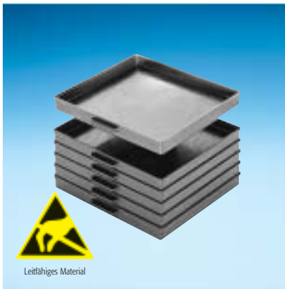
Art.-Nr. V 1-1/16-6-10 als Stapelbehälter
