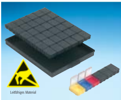
Art.-Nr. 36 SMD-Boxen N3 genau passend in A 1-4/16-6-10 Innenmaß 340 x 250 x 22
