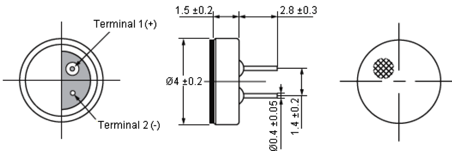
Dimensions : Millimetres
