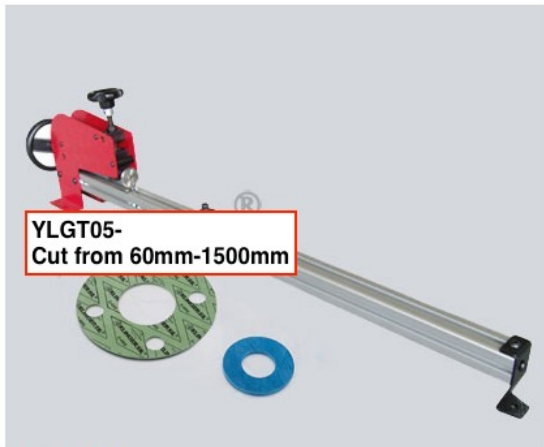
名 称：新型垫片切割器 产品型号：YLGT05-60-1500
