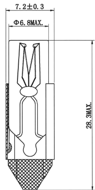
Dimensions : Millimetres
