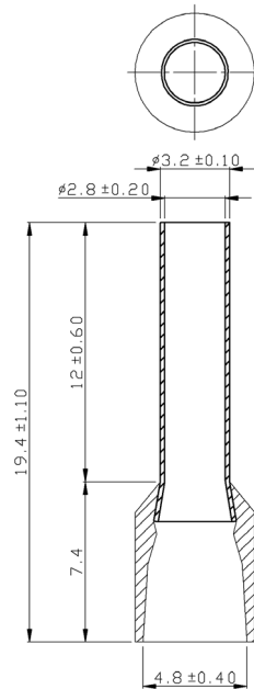
Dimensions : Millimetres
