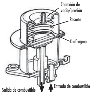
FIGURA 6: REGULADOR DE PRESIÓN
