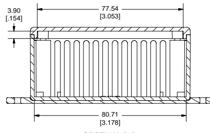
SECTION D-D
