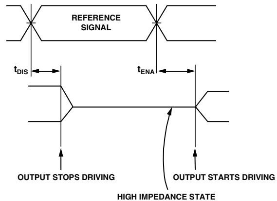
Figure 27. Output Enable/Disable
