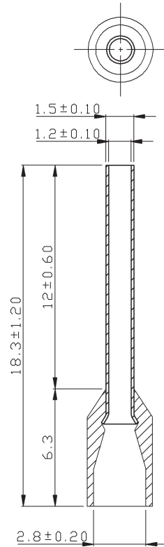
Dimensions : Millimetres
