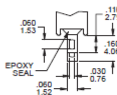
M1 Solder lug
