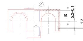
Section D M 3:1
