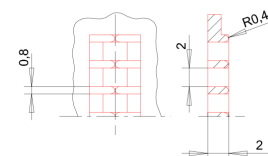
Note X M 3:1
