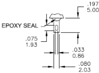
SOLDER LUG
