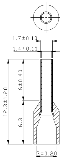
Dimensions : Millimetres
