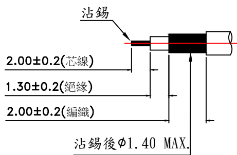
SMA Cable Stripping Dim.
