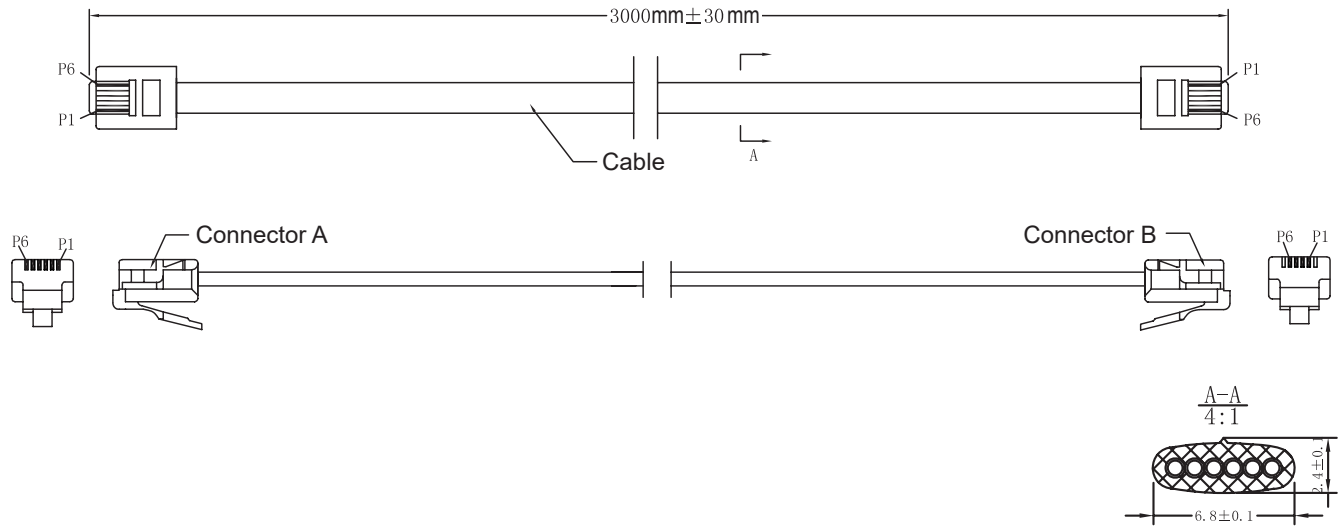
Dimensions : Millimetres
