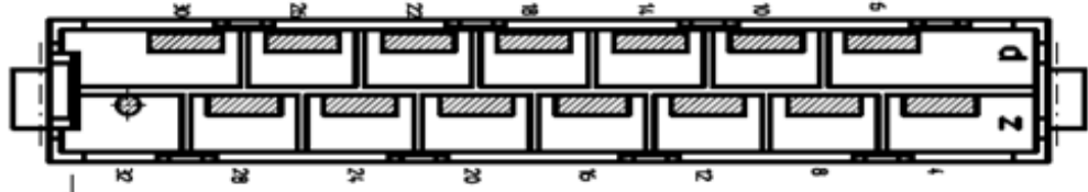
Bestückungsplan / contact layout
