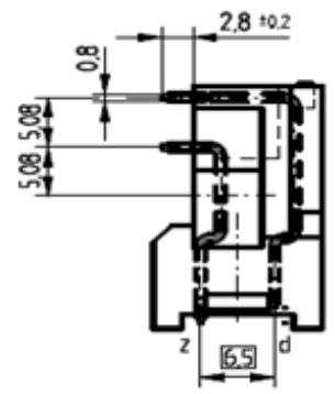
Bestückungsplan / contact layout
