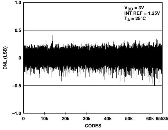
Figure 16. DNL AD5669R-1—Internal Reference
